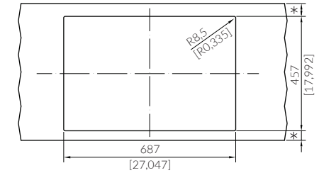
LUXOR COMPACT SI71 A - LUXOR COMPACT SI71 STA
