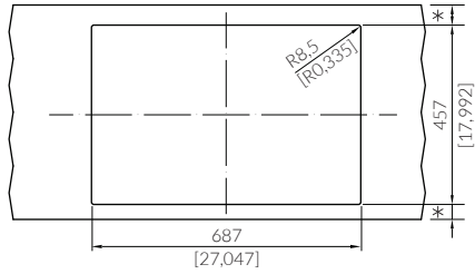
QUADRA MAX Q71 A
