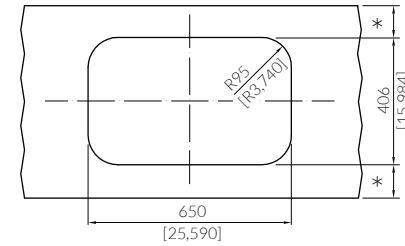
ZARA D84 A
