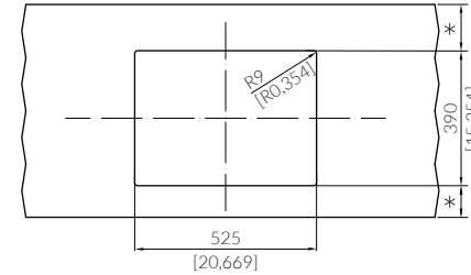
LUXOR MINI SI55 A
